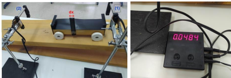
Εικόνα 3. Μέτρηση με το σύστημα φωτοπυλών
